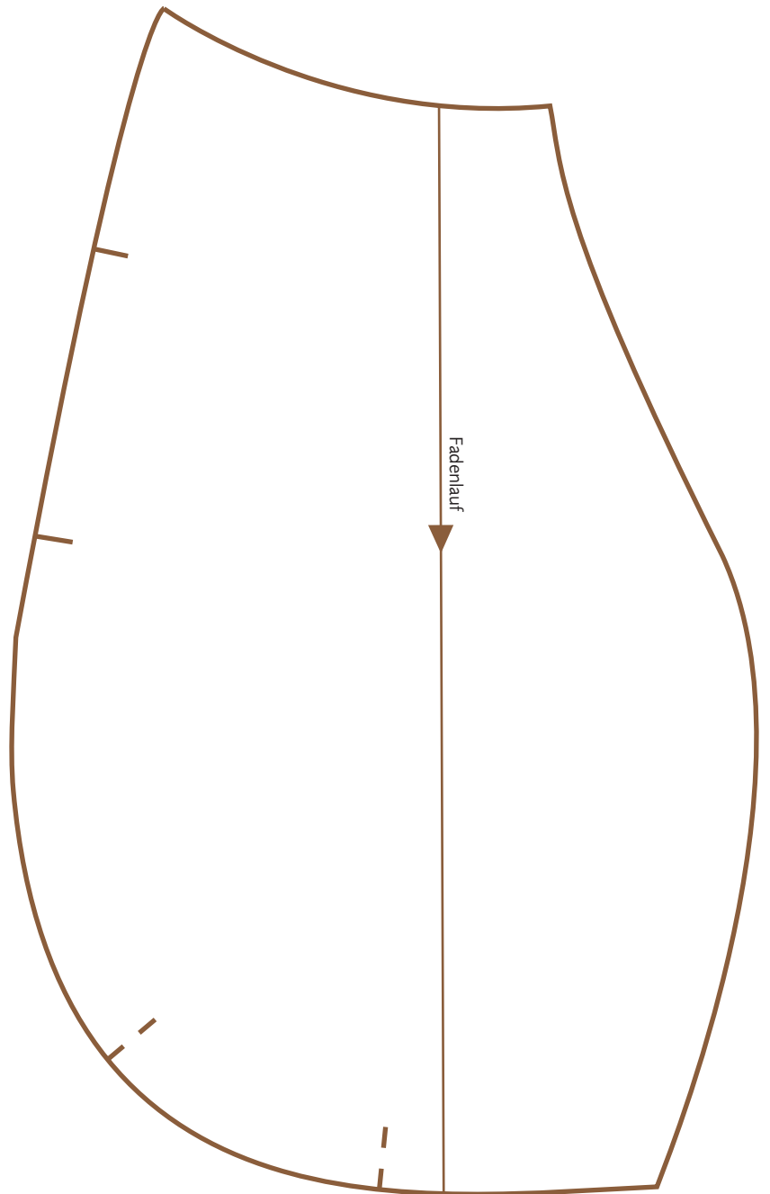
BAUCH 2 x Fell in Beige — Position Arm - - - Position Bein inkl. 7 mm Nahtzugabe
